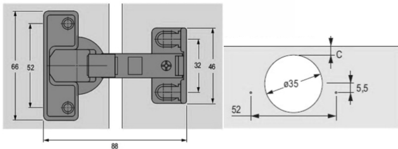
ГАБАРИТЫ МЕБЕЛЬНОГО ФРОНТА И ХОЛОДИЛЬНИКА
