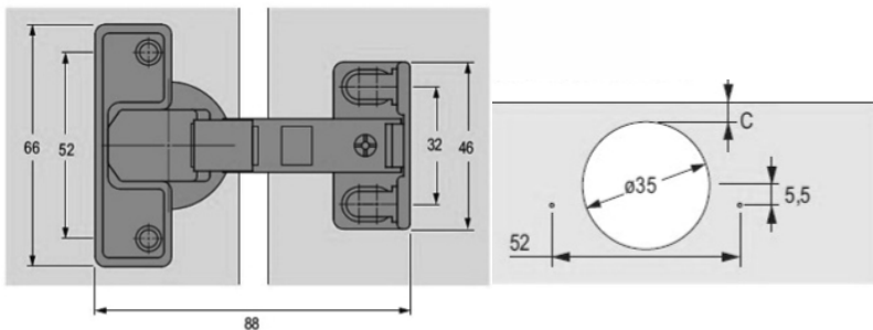
ЖИҢАЗ ФРОНТЫ МЕН ТОҢАЗЫТҚЫШТЫҢ ӨЛШЕМДЕРІ
